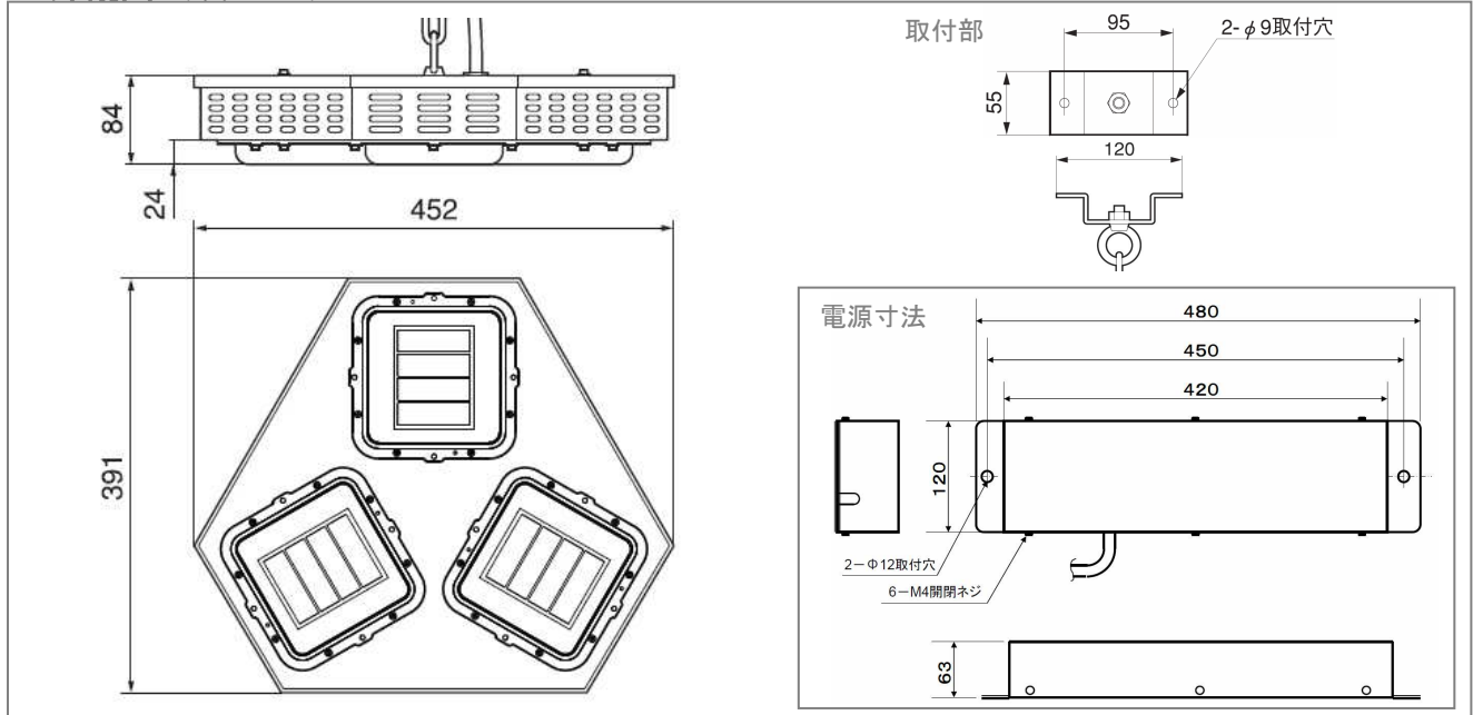
■外観図 (単位:mm)
